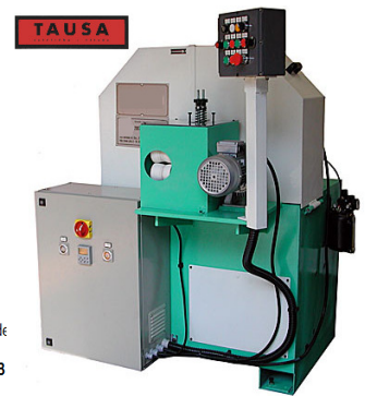
Esmeriladora para elementos cuadrados con un lado máximo de 30mm (OPCIONAL) El disco A permanece bloqueado, rotan las bandas abrasivas B
